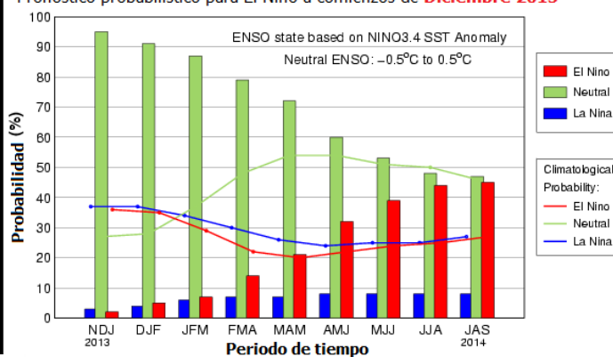
Pronóstico probabilístico para El Niño a comienzos de Diciembre 2013
