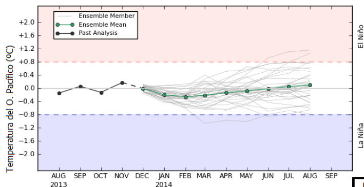
POAMA Promedio mensual NIÑO34 - Pronóstico desde el 1 de Dic 2013
